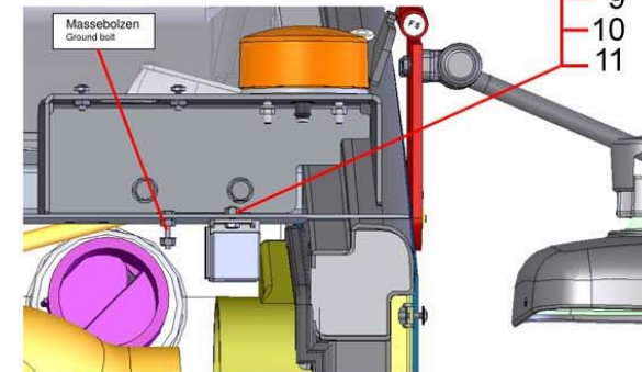
Ansicht Dach von oben Top view roof
